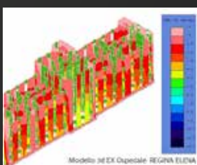
MODELLO 3D EX-OSPEDALE REGINA ELENA, ROMA
